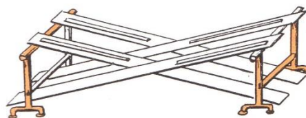
Pracovní stůl pro natírání dveřních křídél
